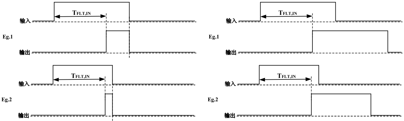
图 8 典型输入滤波 (左) 增强型输入滤波 (右)
