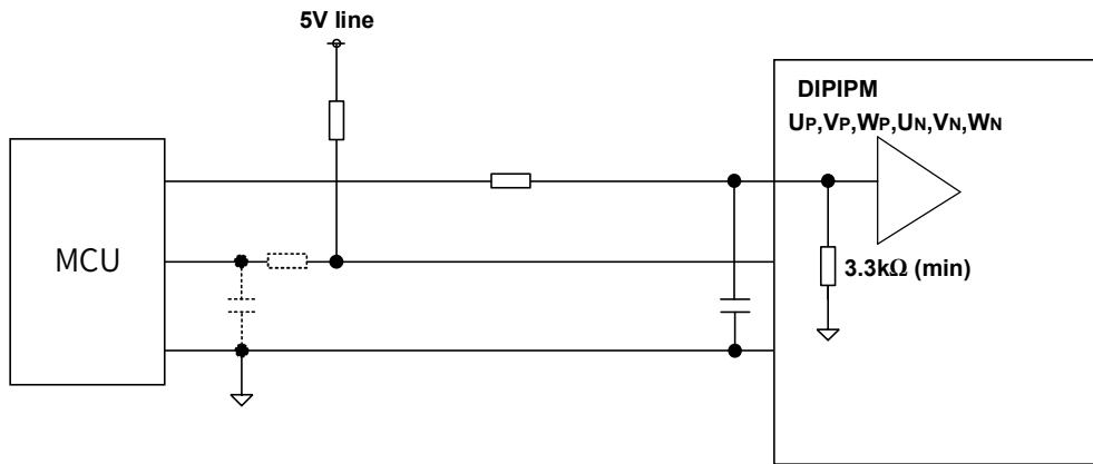
图 12 推荐的 MCU 输入输出接口电路
