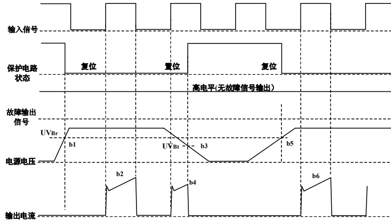
图 10 欠压保护时序图 (高侧)
