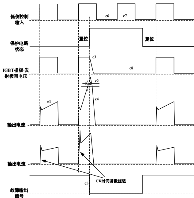
图 11 短路电流保护时序图 (只适合于低侧)
