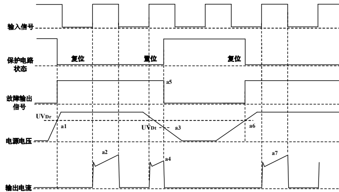
图 9 欠压保护时序图 (低侧)
