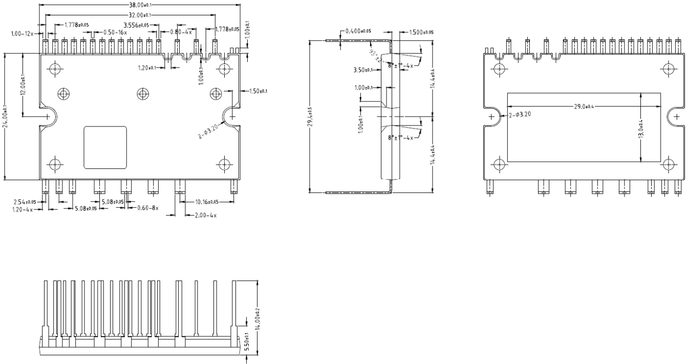
图 15 外型封装图
