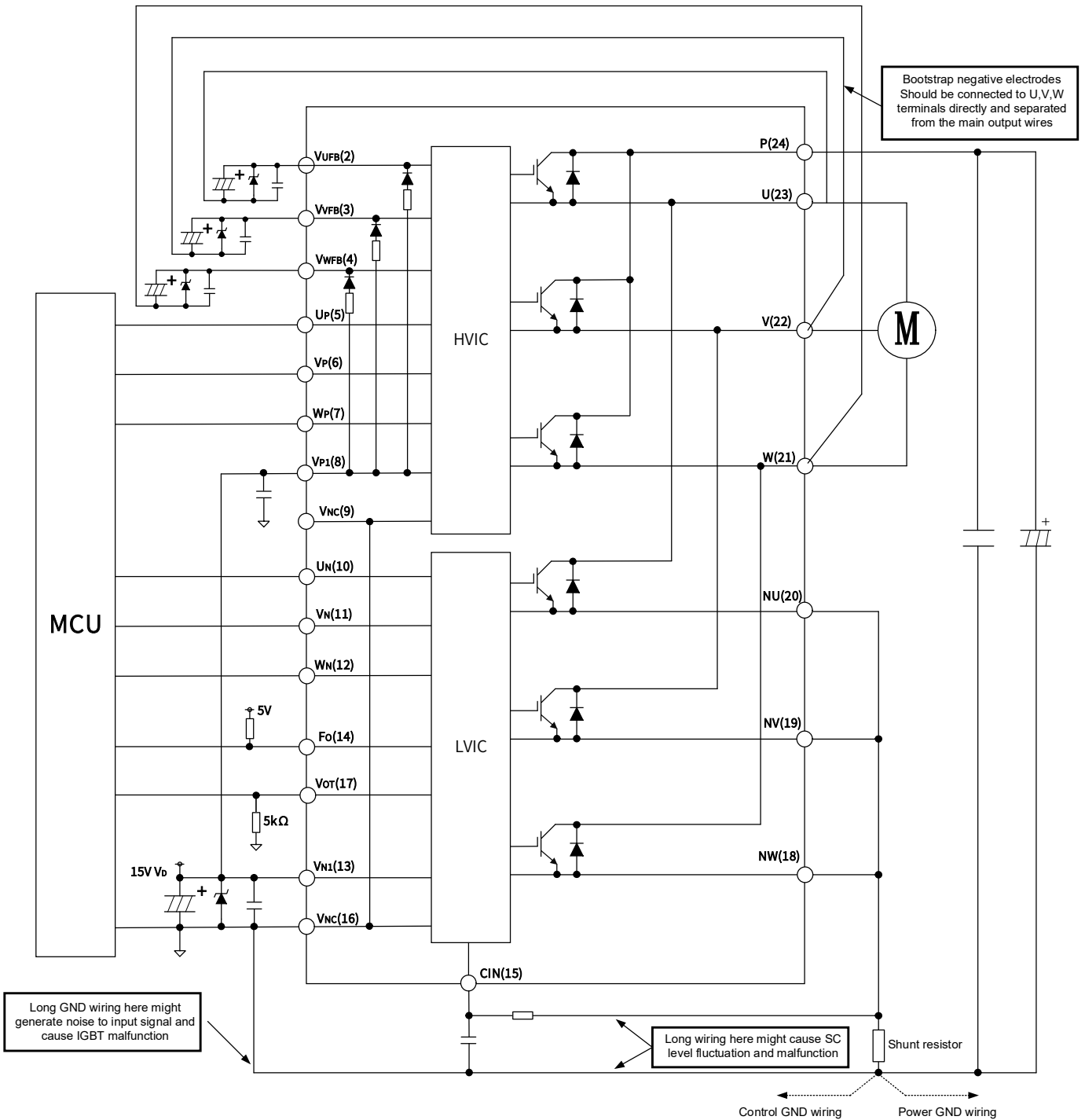
图 14 典型应用路
