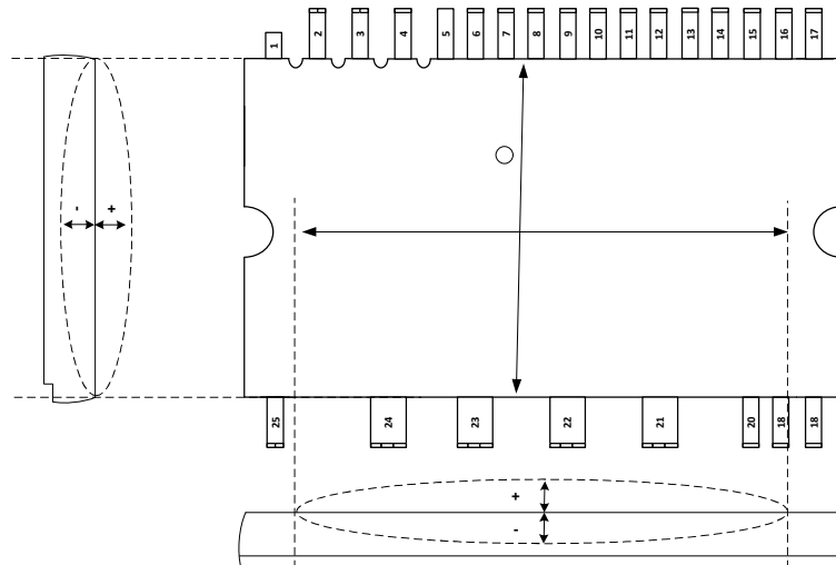
图 7 平面检测位置
