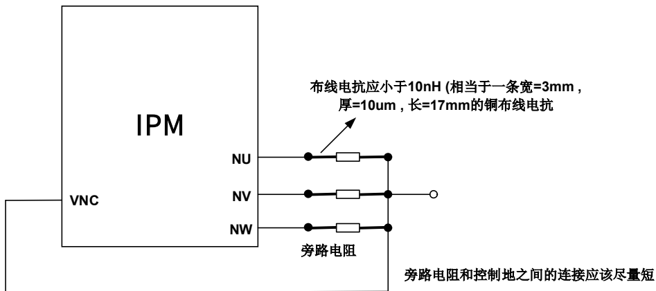
图 13 旁路电阻接线注意事项
