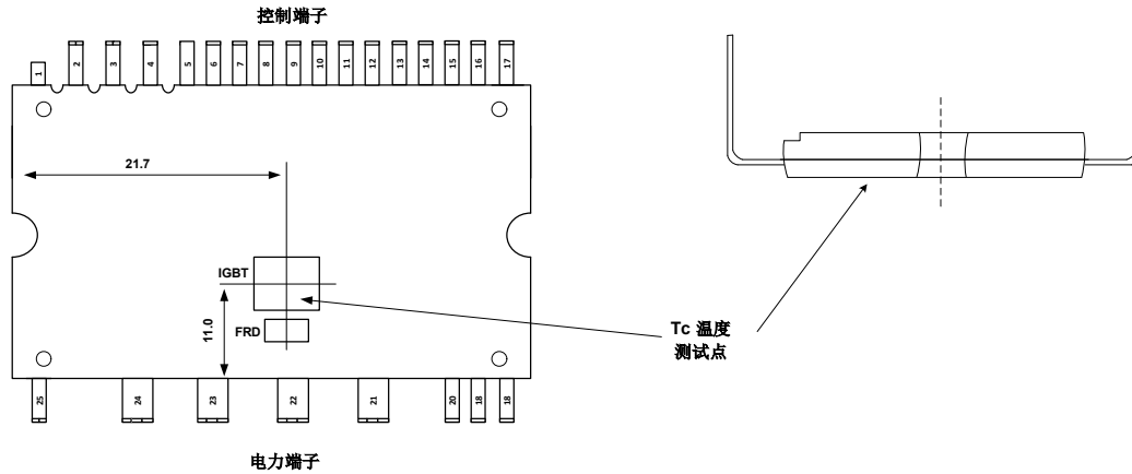
图 3 壳温测试点
